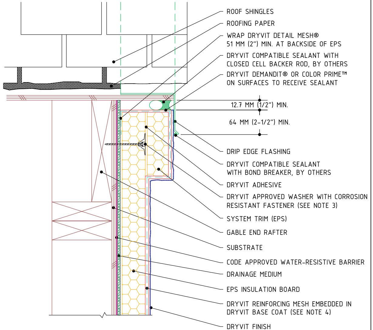
SECTION A-A
